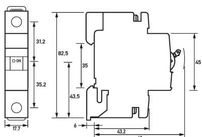
Maßzeichnung Leitungsschutzschalter DLS 6i Do2-1
