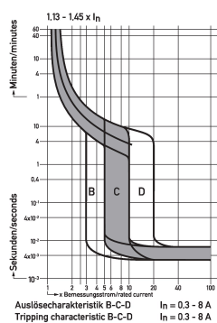
Diagramme Leitungsschutzschalter DLS 6i Co,5-4
