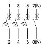
Schaltungsbeispiel Leitungsschutzschalter DLS 6i C1,6-3+N
