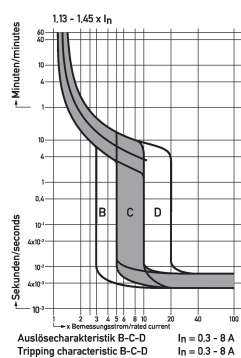
Diagramme Leitungsschutzschalter DLS 6i Co,8-3+N
