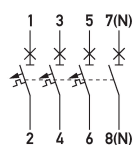
Schaltungsbeispiel Leitungsschutzschalter DLS 6i Co,8-3+N
