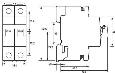
Maßzeichnung Leitungsschutzschalter DLS 6i Co,8-2
