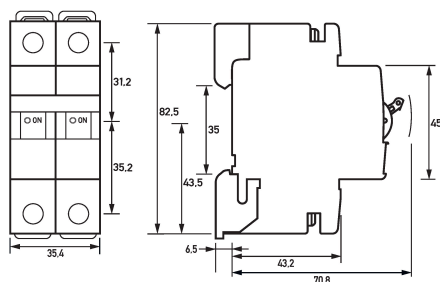
Maßzeichnung Leitungsschutzschalter DLS 6i C5-1+N
