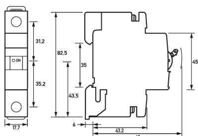
Maßzeichnung Leitungsschutzschalter DLS 6i Co,3-1
