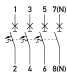
Schaltungsbeispiel Leitungsschutzschalter DLS 6i B4-3+N
