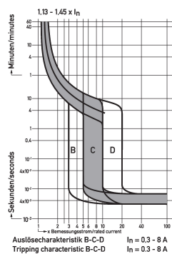
Diagramme Leitungsschutzschalter DLS 6i B 3,5-3+N
