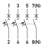
Schaltungsbeispiel Leitungsschutzschalter DLS 6i B 3 -3+N
