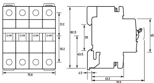
Maßzeichnung Leitungsschutzschalter DLS 6i B2,5-3+N
