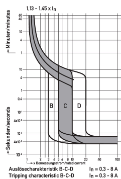
Diagramme Leitungsschutzschalter DLS 6i B2-3+N
