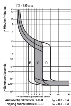
Diagramme Leitungsschutzschalter DLS 6i B1-3+N
