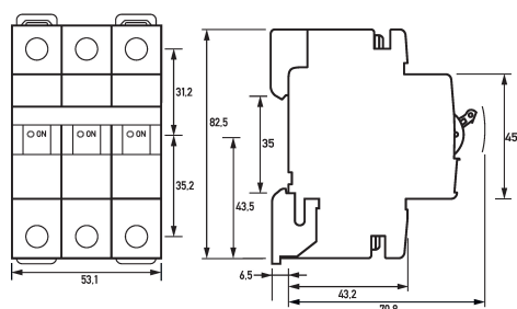
Maßzeichnung Leitungsschutzschalter DLS 6i B 3,5 -3
