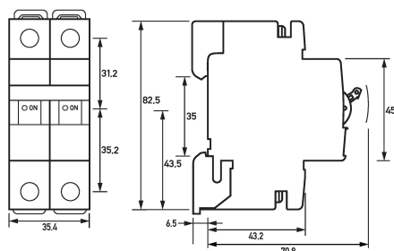
Maßzeichnung Leitungsschutzschalter DLS 6i B5-2
