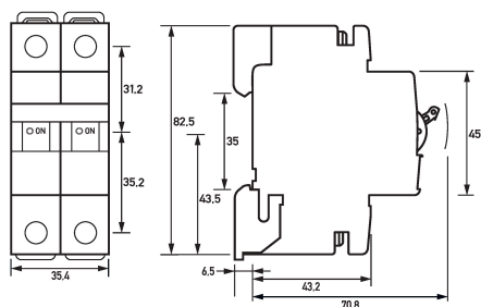
Maßzeichnung Leitungsschutzschalter DLS 6i Bo1-1+N
