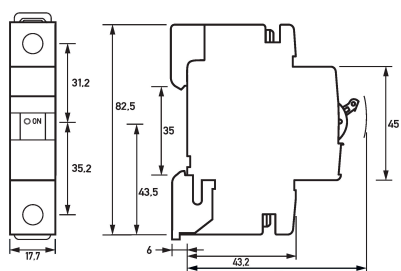
Maßzeichnung Leitungsschutzschalter DLS 6i Bo2,5-1
