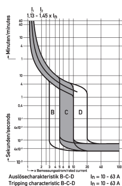
Diagramme Leitungsschutzschalter DLS 6h C25-4
