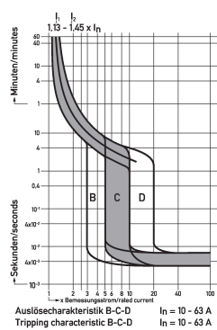
Diagramme Leitungsschutzschalter DLS 6h C20-4
