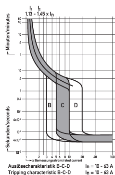
Diagramme Leitungsschutzschalter DLS 6h C16-4
