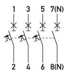
Schaltungsbeispiel Leitungsschutzschalter DLS 6h C16-3+N
