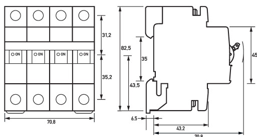
Maßzeichnung Leitungsschutzschalter DLS 6h C13-3+N
