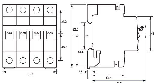
Maßzeichnung Leitungsschutzschalter DLS 6h C10-3+N
