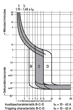
Diagramme Leitungsschutzschalter DLS 6h C10-3+N
