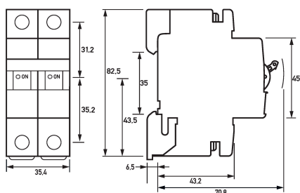
Maßzeichnung Leitungsschutzschalter DLS 6h C13-2
