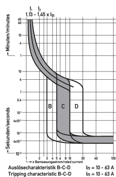
Diagramme Leitungsschutzschalter DLS 6h C13-2
