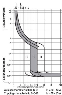
Diagramme Leitungsschutzschalter DLS 6h C13-1+N
