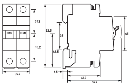
Maßzeichnung Leitungsschutzschalter DLS 6h C13-1+N
