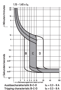
Diagramme Leitungsschutzschalter DLS 6h C6-1+N
