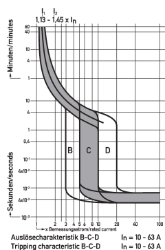
Diagramme Leitungsschutzschalter DLS 6h B20-4
