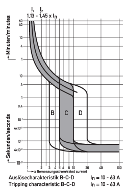
Diagramme Leitungsschutzschalter DLS 6h B10-4
