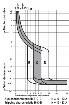
Diagramme Leitungsschutzschalter DLS 6h B20-3+N
