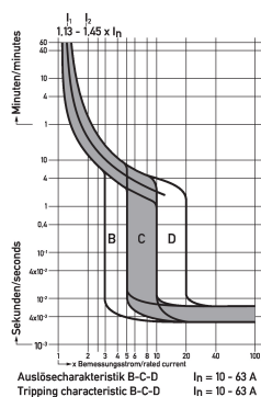
Diagramme Leitungsschutzschalter DLS 6h B10-3+N
