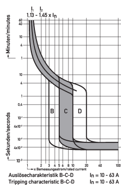
Diagramme Leitungsschutzschalter DLS 6h B25-2
