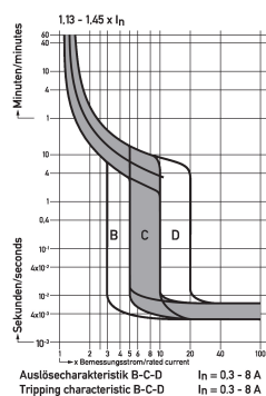
Diagramme Leitungsschutzschalter DLS 6h B6-2
