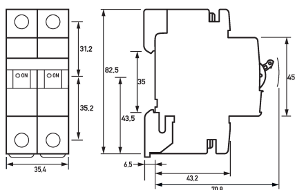
Maßzeichnung Leitungsschutzschalter DLS 6h B25-1+N
