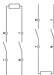
Schaltungsbeispiel Leitungsschutzschalter DLS 6hdc C25-2
