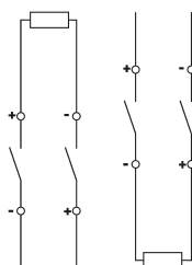
Schaltungsbeispiel Leitungsschutzschalter DLS 6hdc C4-2
