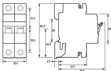
Maßzeichnung Leitungsschutzschalter DLS 6hdc B32-2
