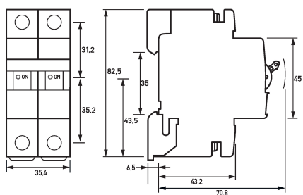
Maßzeichnung Leitungsschutzschalter DLS 6hdc B25-2
