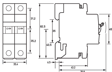
Maßzeichnung Leitungsschutzschalter DLS 6hdc B20-2
