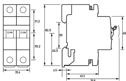
Maßzeichnung Leitungsschutzschalter DLS 6hdc B16-2
