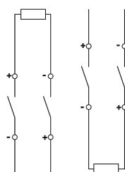
Schaltungsbeispiel Leitungsschutzschalter DLS 6hdc B16-2
