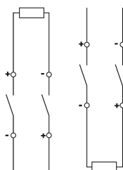
Schaltungsbeispiel Leitungsschutzschalter DLS 6hdc B2-2
