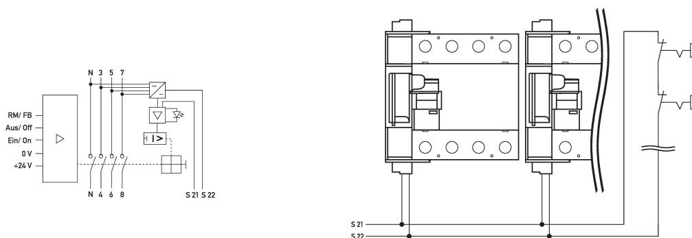
Schaltungsbeispiel Lasttrennschalter DHS 4-125 FANA24DC
