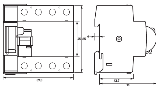
Maßzeichnung Lasttrennschalter DHS 4-125 FANA24DC
