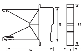
Maßzeichnung Distanzstücke DHDS
