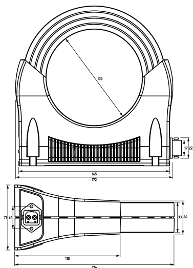
Maßzeichnung Messwandler DRCA 1 CT 105
