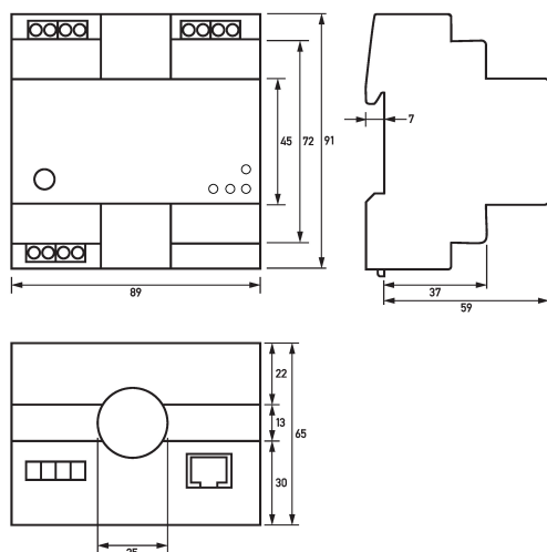
Maßzeichnung Differenzstrommonitore e.Guard RCM F 025
