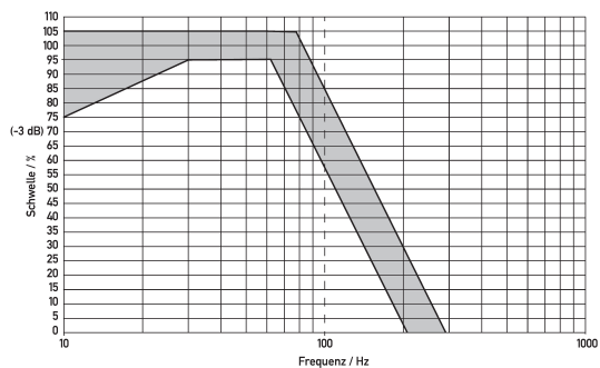
Diagramme Differenzstrommonitore e.Guard RCM F 025
