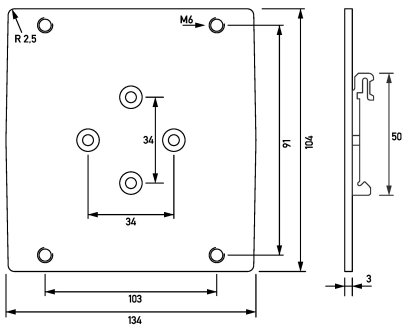
Maßzeichnung Tragschienenadapter RCM Mount B 070
