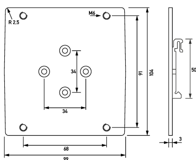
Maßzeichnung Tragschienenadapter RCM Mount B 035
