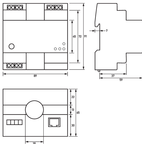
Maßzeichnung Differenzstrommonitore e.Guard RCM B 025
