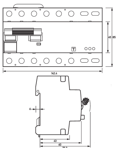
Maßzeichnung Ortsveränderliche Fehlerstromschutzeinrichtungen DPRCD-M2
