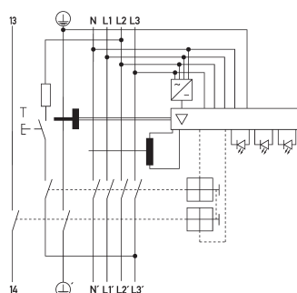
Schaltungsbeispiel Ortsveränderliche Fehlerstromschutzeinrichtungen DPRCD-M2
