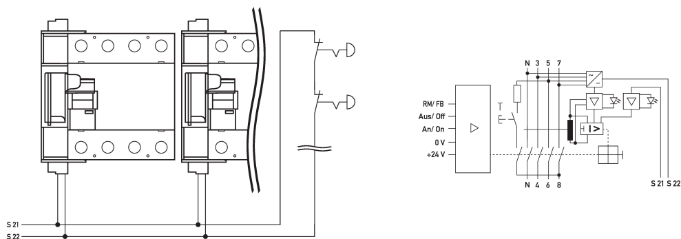
Schaltungsbeispiel Fehlerstromschutzschalter DFS 4 125-4/0,03-B SK FANA24DC
