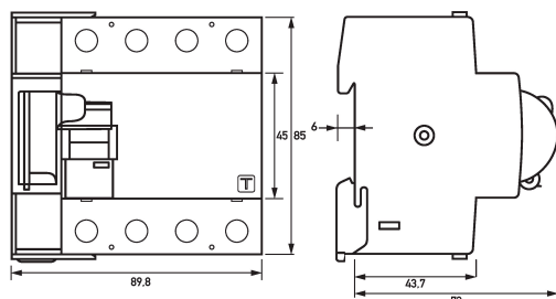
Maßzeichnung Fehlerstromschutzschalter DFS 4 125-4/0,03-B SK FANA24DC
