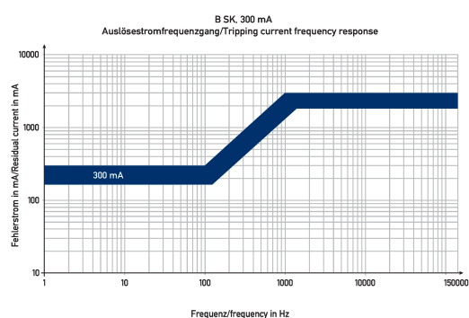
Diagramme Fehlerstromschutzschalter DFS 4 080-4/0,30-B SK MI
