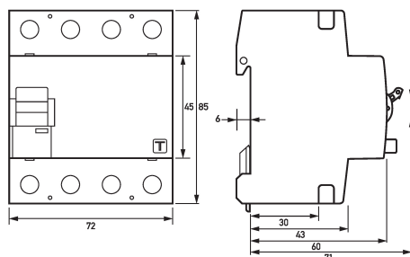
Maßzeichnung Fehlerstromschutzschalter DFS 4 080-4/0,30-B SK MI
