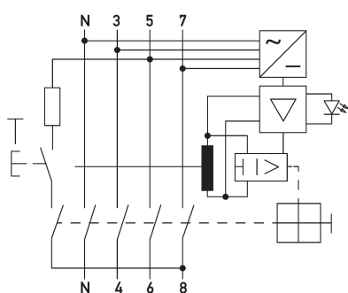
Schaltungsbeispiel Fehlerstromschutzschalter DFS 4 080-4/0,30-B SK MI
